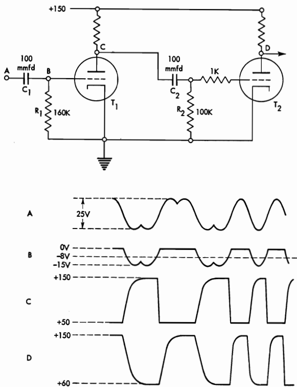
Figure II-25. Shaping Amplifier SA 506
